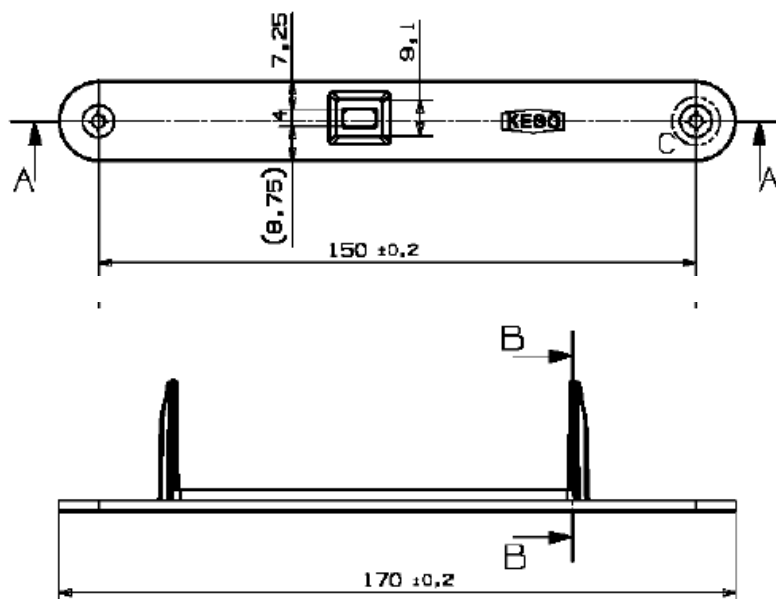
Stulpblende kurz
